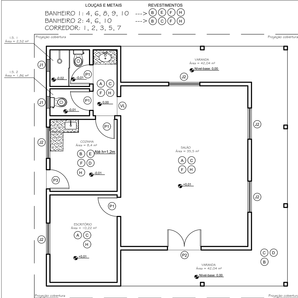
NUMEAR - Planta de esquadrias e revestimentos Esc. 1:75
