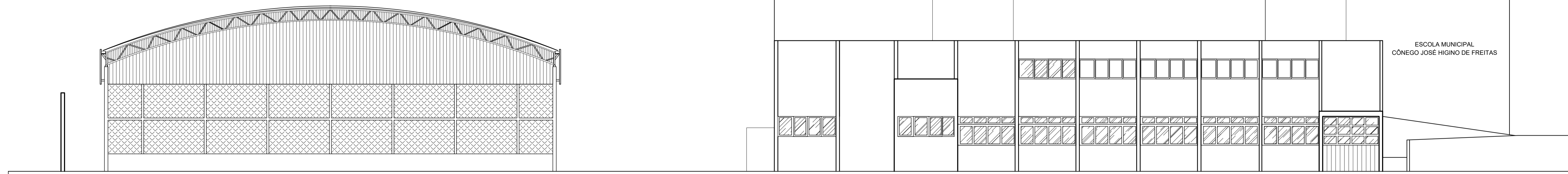
20 FACHADA COM IMPLANÇÃO DA QUADRA Esc. 1:120
